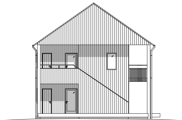
TYP A - FASAD NORR
