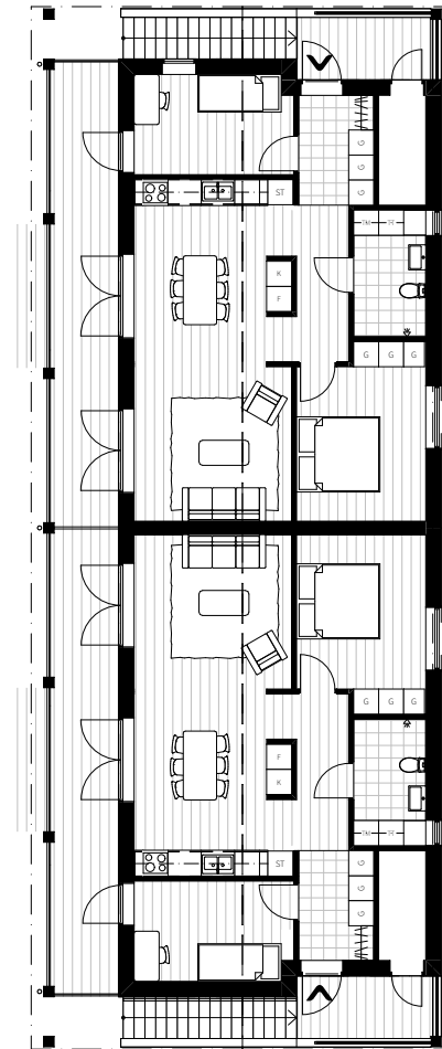
TYP A - PLAN 2
